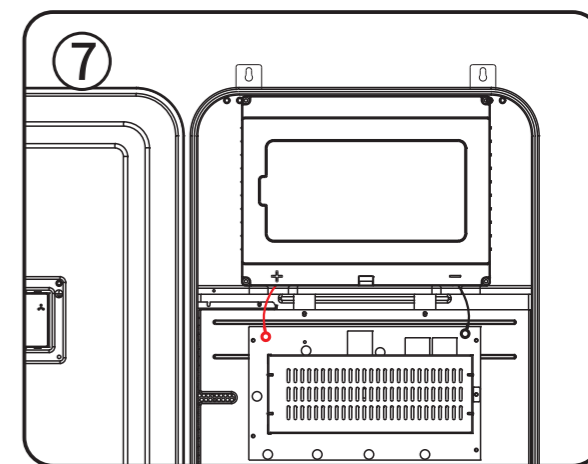
将备用电源装入箱内,注意备用电源需倒置安装,并且备用电源的正负极不得接反
