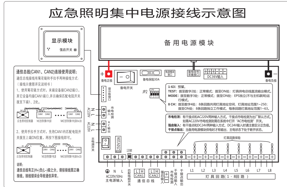
500W应急照明集中电源接线示意图 图4.1
