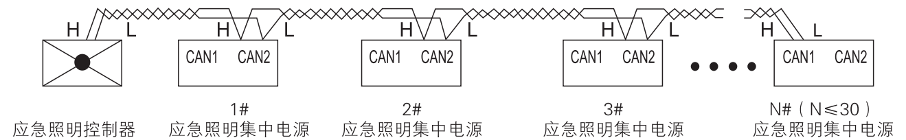
菊花链连接方式示意图（图2）
