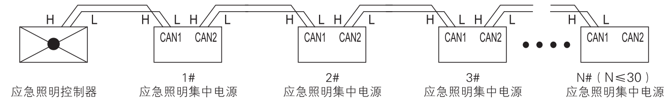
手拉手连接方式示意图（图1）
